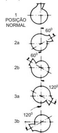
POSIÇÕES DA BOCA DE RECÁLQUE (1) (visto pelo lado do acionamento)
